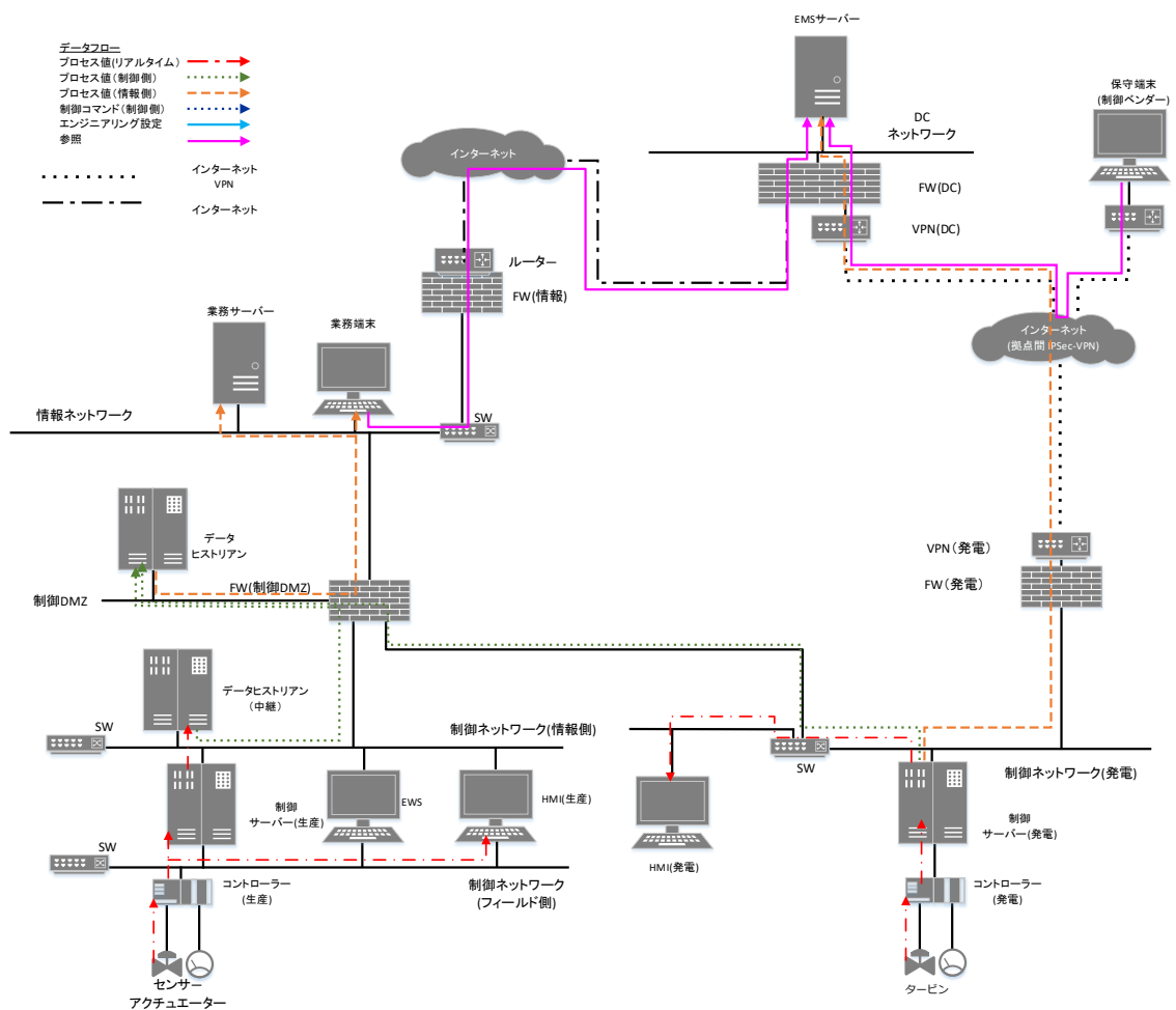
図 2-5 データフロー図(プロセスデータ・参照)
