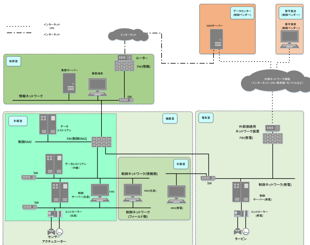
図 1-6 分析対象システムの構成図（外部ネットワーク接続の詳細は不明）
