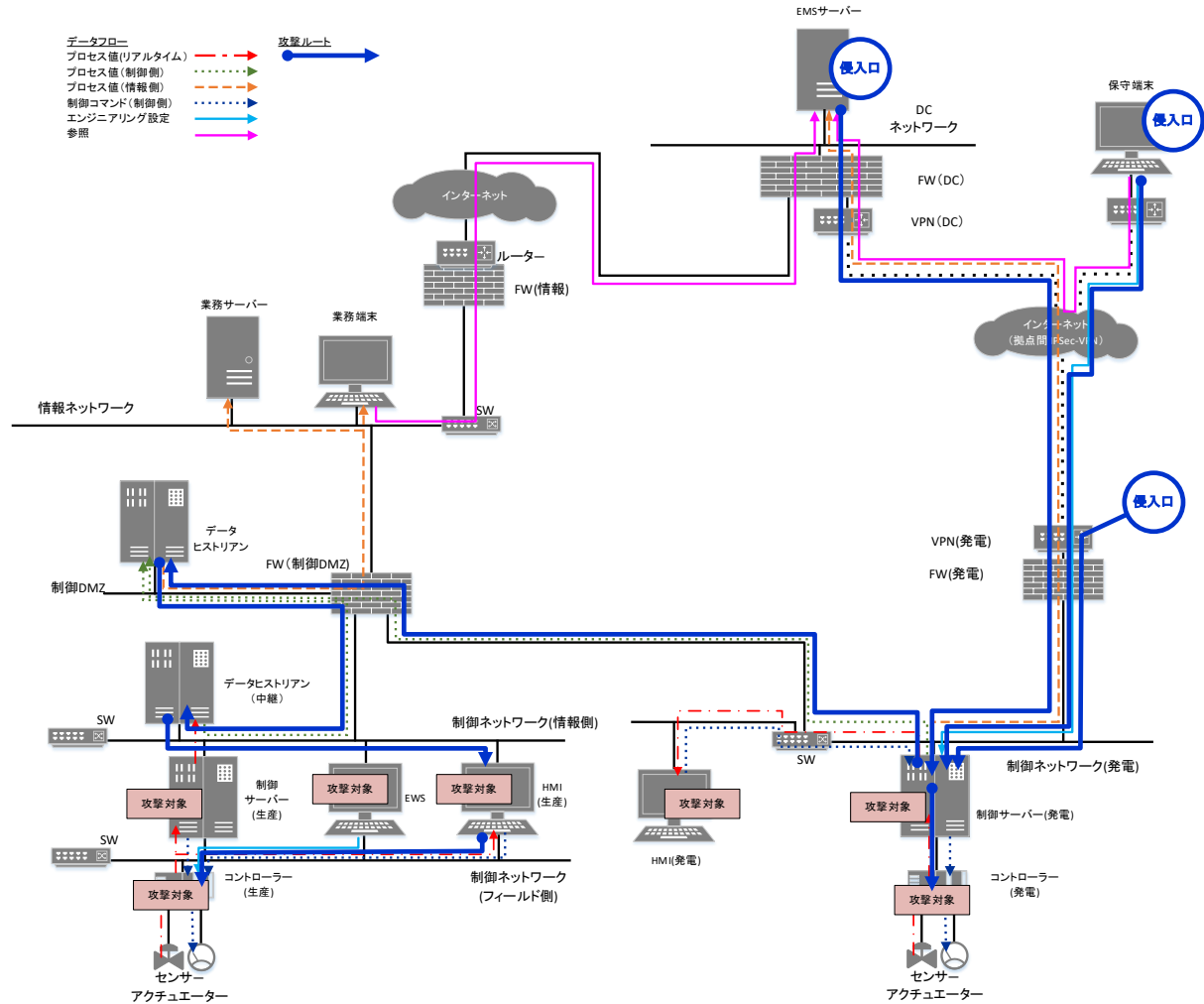
図 4-3 攻撃ルート図
