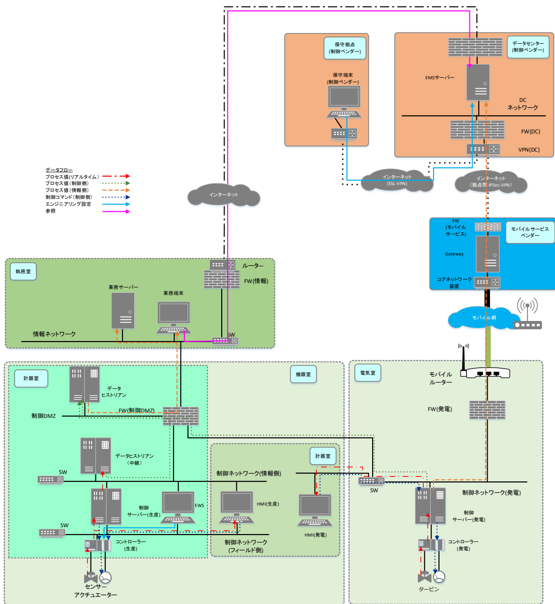
図 C-3 データフロー
