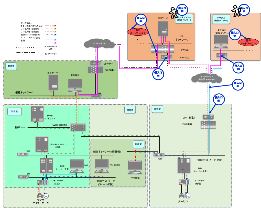
図 4-2 侵入口の候補
