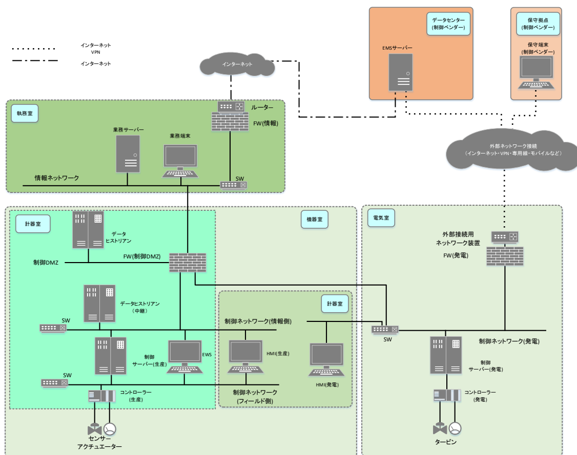
図 2-2 システム構成図
