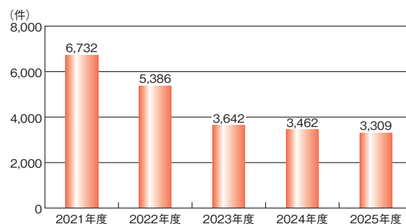
■ 図 1-1-19 DDoS 攻撃の検出件数 (2021～2025 年度)
