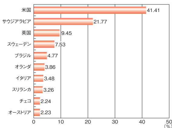
■ 図 1-1-4 DDoS トラフィックの攻撃対象国上位 10 か国 (2025 年) (出典)DigiCert, Inc.「UltraDDoS Protect Annual Distributed Denial-of-Service Analysis, January–December 2025 *14 」を基に IPA が編集
