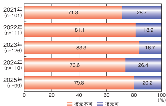
■ 図 1-1-18 ランサムウェア感染後、取得していたバックアップからの復元結果 (2021～2025 年)
