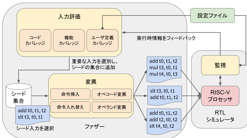
図 4: ファザーの全体像
