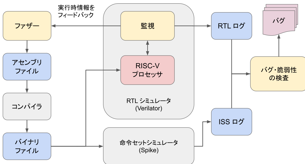
図 3: MicroFuzz の全体像
