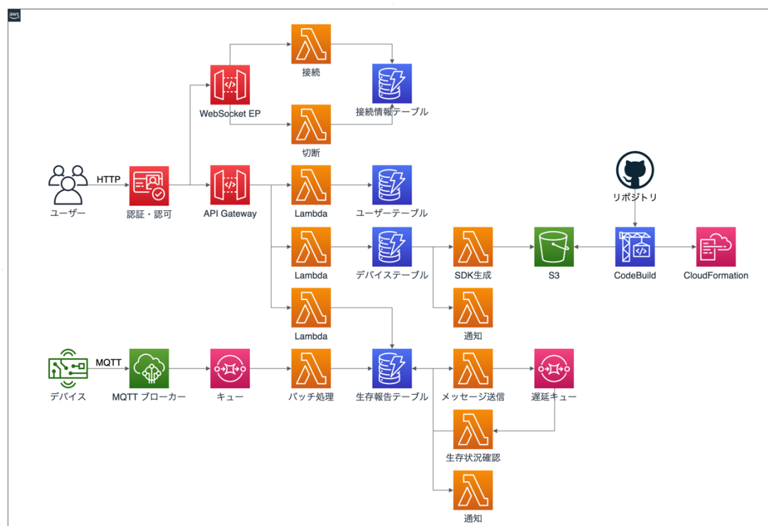
図 4. バックエンドのアーキテクチャ図
