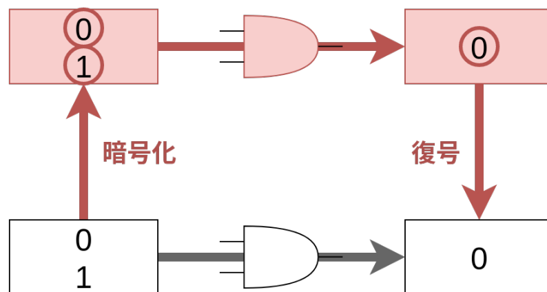
図 1: 準同型暗号
