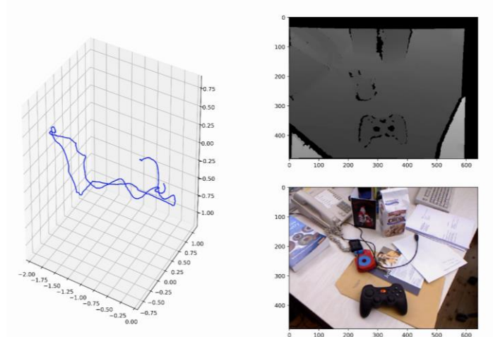
図 2. DVO によるカメラの移動量の推定結果
