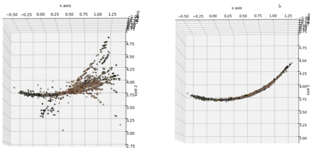
図 3. Bundle Adjustment を用いた誤差の修正結果
