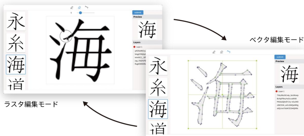
図 3. DeepGlyph のインタフェース (修正 UI)
