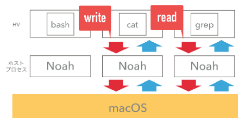
図 4 cat file | grep mitou の動作
