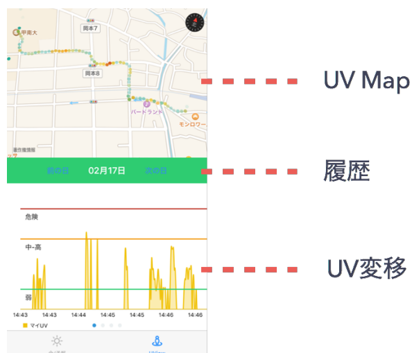
図 6 UView 画面
