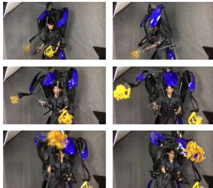
図 2 パンチ動作
