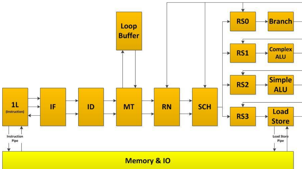
図 1 MIST1032SA のパイプライン
