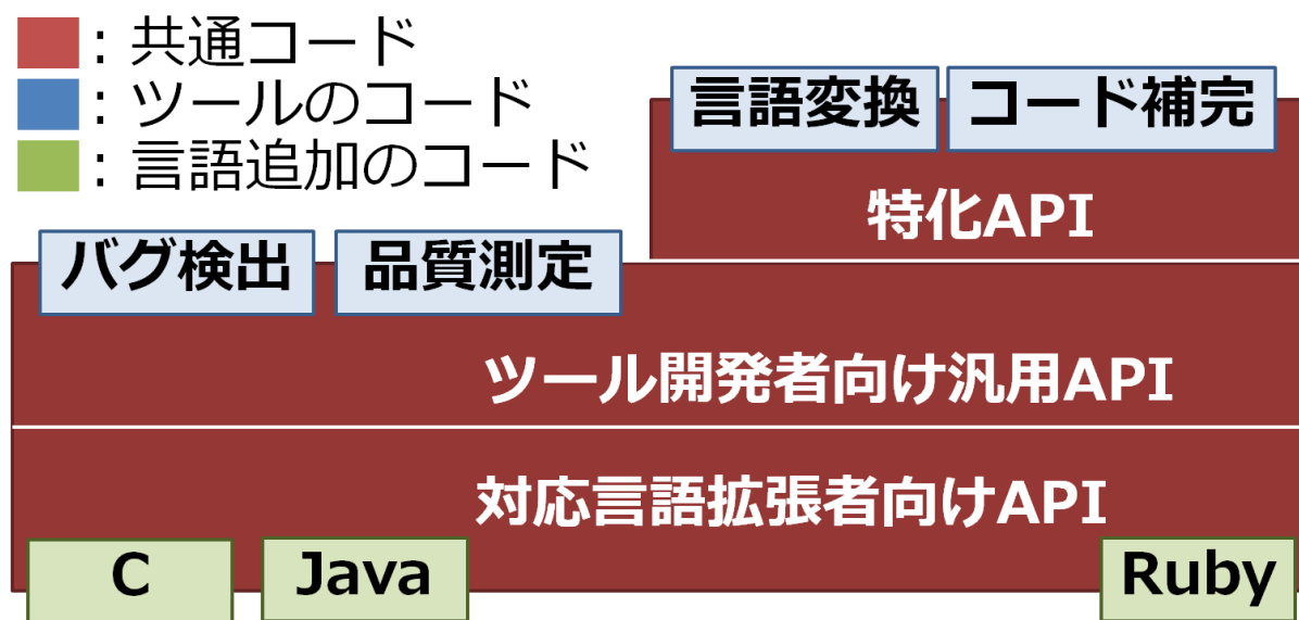
図 2. UNICOEN のアーキテクチャ
