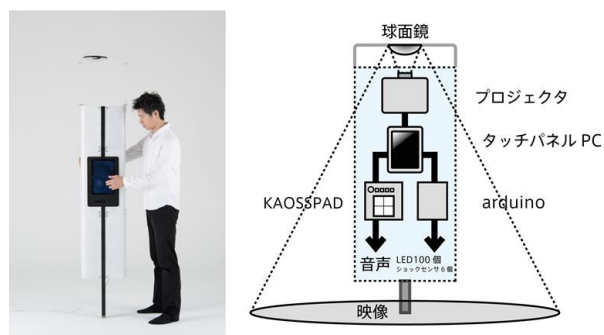
図 2. mirage00 の構成
