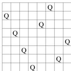
図 1. N-Queens Problem
