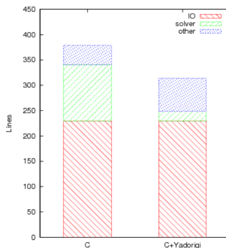
図 2. N-Queens ソルバの比較
