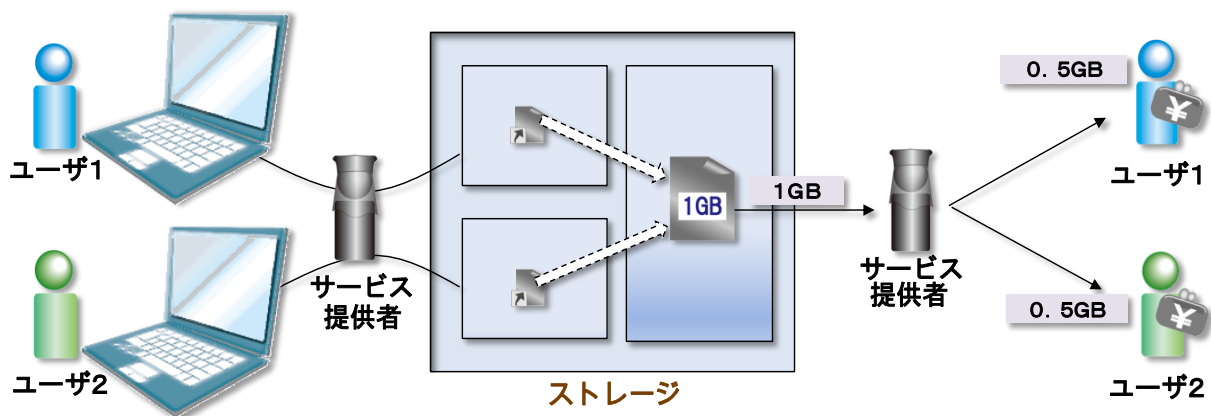
図 2 ファイルサイズ分配機能
