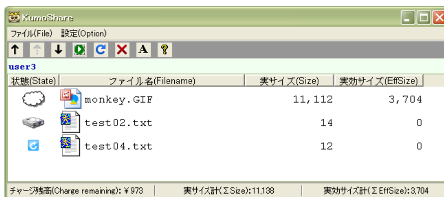
図 4 選択的同期機能
