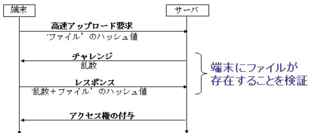
図 3 検証機能付き高速アップロード機能
