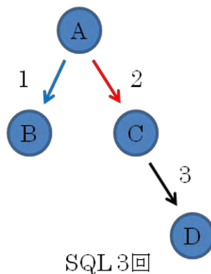
図1: 循環参照がない場合のマーキング SQL の最適な発行順序。図中の円で表された A、B、C、D はそれぞれ DB 中のテーブルを意味し、矢印がマーキング SQL を意味する。
