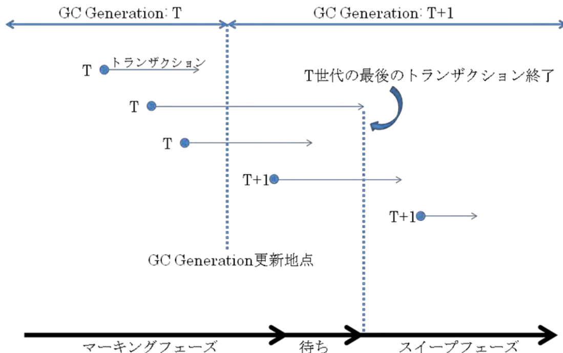
図2:DB で湯浅式 GC を実現するために必要なトランザクションの状態と、マークフェーズとスイープフェーズを実行する時期との関係を表した。
