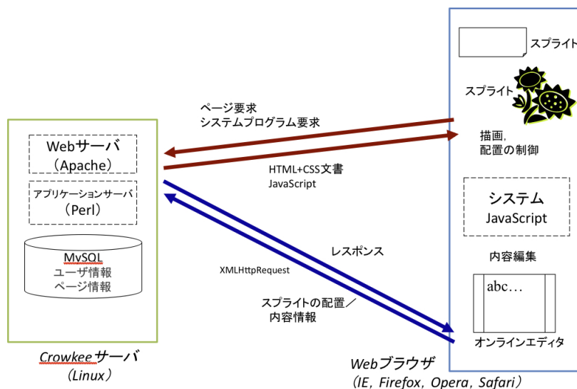
図 2：システム構成図
