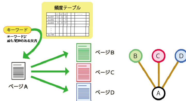
図4 木構造の生成の流れ
