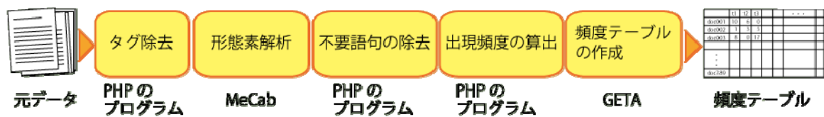
図3 単語出頻度テーブルの生成
