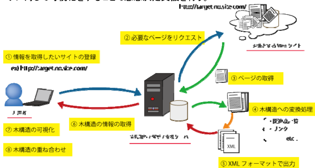
図1 システム全体の流れ
