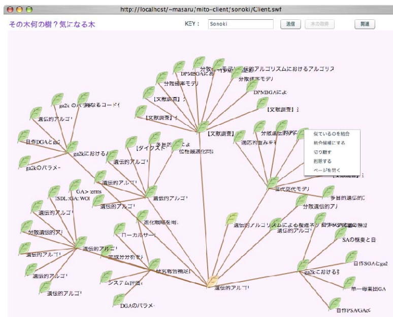
図5 クライアントアプリケーションの実行例
