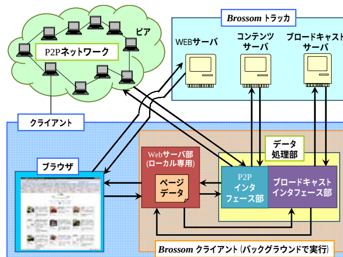
図5: P2P ストリーミング型放送 Brossom の構成
