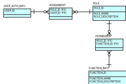
図 3.2.1「ER 図」
