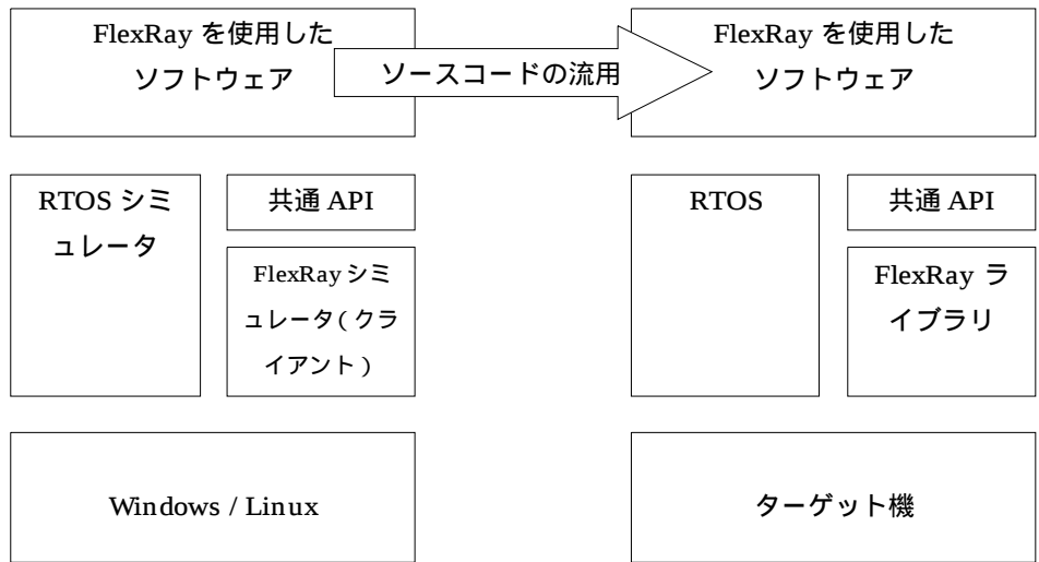
図2 シミュレーション開発後 の実機上での開発
