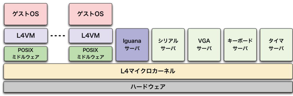
図 1：L4VM システム構成図
