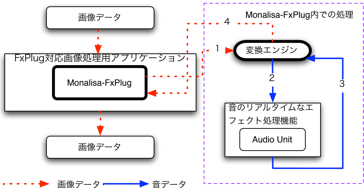
図6：Monalisa-FxPlugを利用した処理
