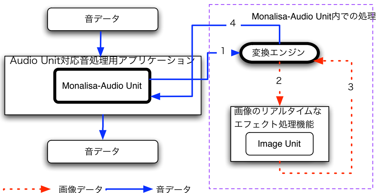
図2：Monalisa-Audio Unitを利用した処理
