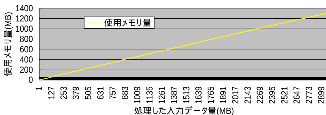
図 1 ヒトゲノム(2.97GB)に対するメモリ使用量
