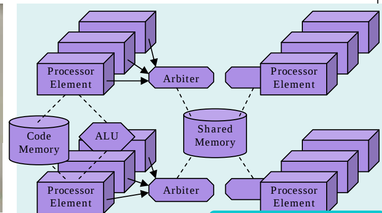
μ SOARSアーキテクチャ
