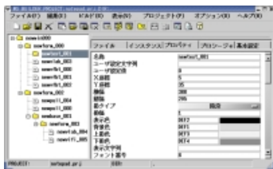
図4 WideStudio アプリケーションビルダー
