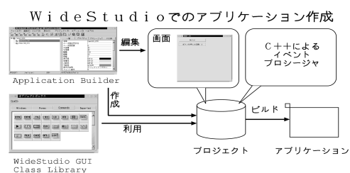
図5 アプリケーション作成の流れ
