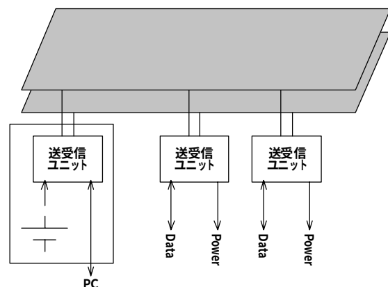
図1. TextileNet システムの構成図
