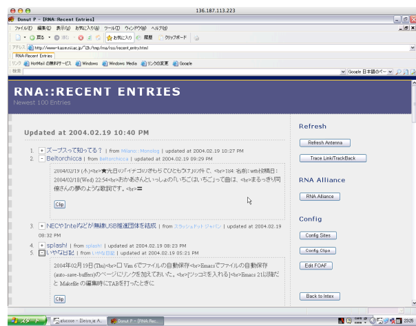
図 1 RNA
