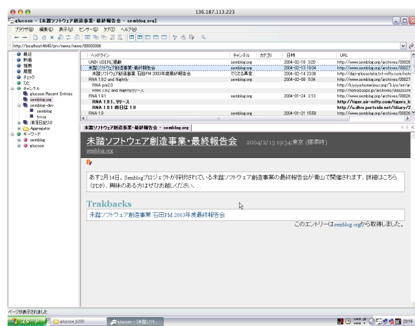
図 2 glucose
