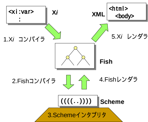
図 2. Xi コンパイラの構成
