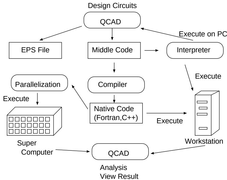
図 1: QCAD の概念図。Windows 上で動作する QCAD で量子回路を設計し、作成した回路は論文用に EPS ファイル、実行用に中間コードで出力される。中間コードはインタプリタで読み込んで実行することができ、結果はそのまま PC で確認できる。インタプリタは独立して動作できるため、ワークステーションなどで、より高速に実行させることもできる。また、中間コードをコンパイルして Fortran や C 言語で出力して実行できる。さらに MPI などを用いた並列化を行い、スーパーコンピュータで実行し、結果を QCAD で解析する。
