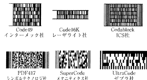
図7: スタック型コードの種類
