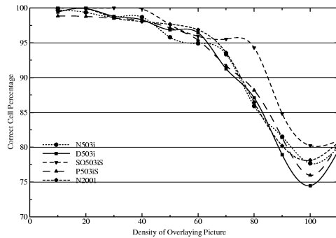
図 30: オーバーレイ画像と認識率の関係
