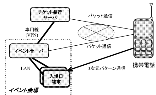
図 2: 電子チケットシステムの概要
