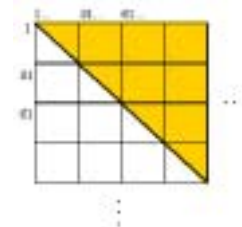
図 3: データ分割 1
