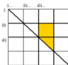
図6: データ分割4
