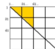
図 4: データ分割 2
