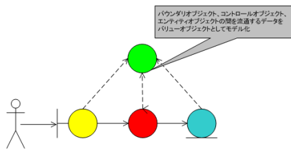
図 19: 分析オブジェクトの使用例
