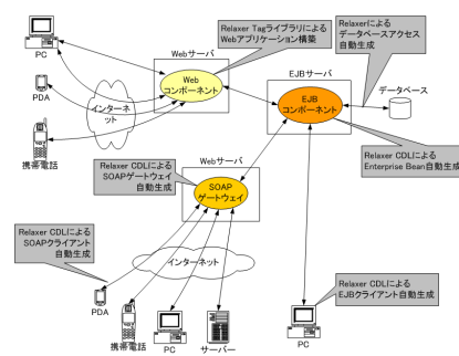
図 5: J2EE における Relaxer
