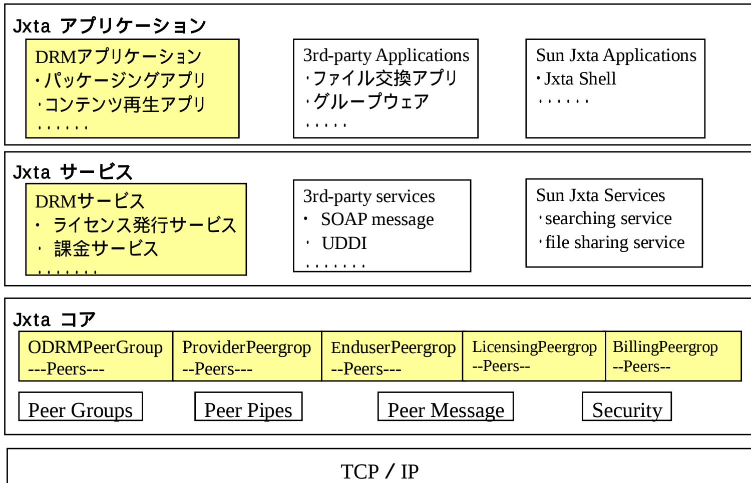
図 2 システムアーキテクチャ
