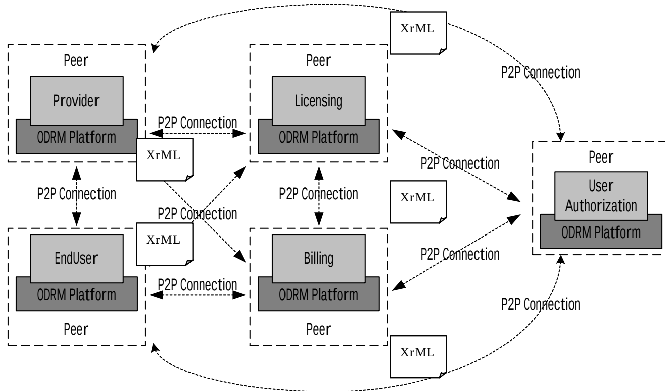
図1 システム動作イメージ
