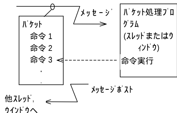
図 2 パケット処理プログラム
