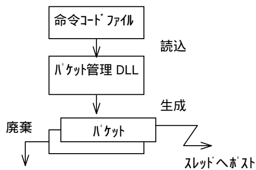
図 3 パケット管理DLL
