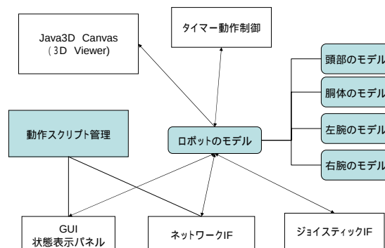
図 3 動作スクリプト編集・動作シミュレータの構成
