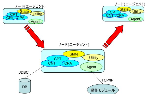
図 9 状態遷移ネットワークの構造
