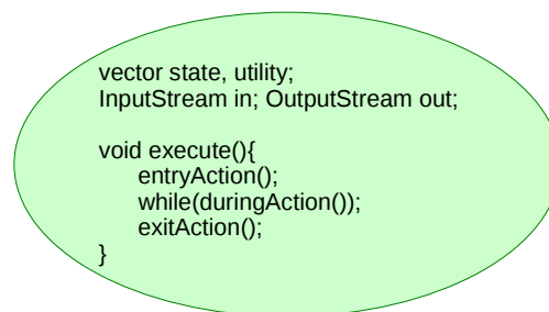
図 10 エージェントの構造
