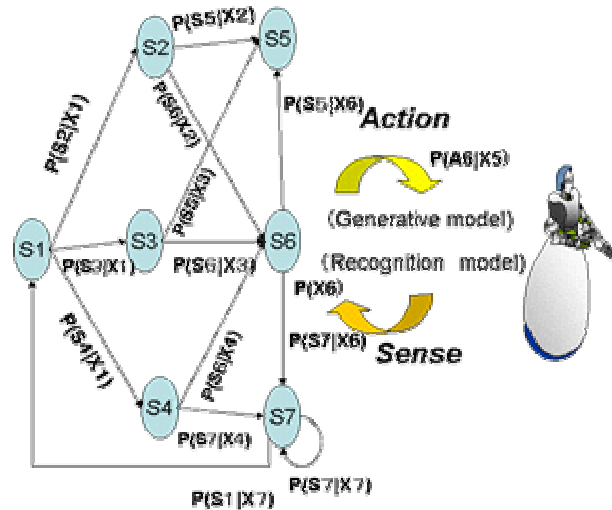
図 8 確率的状態遷移ネットワーク
