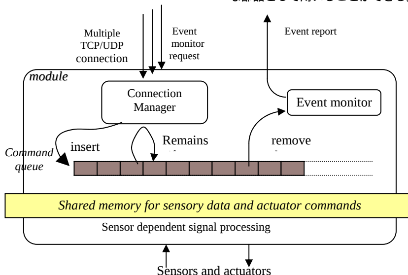
図 2 イベント駆動型ソフトウェアモジュールの構造
