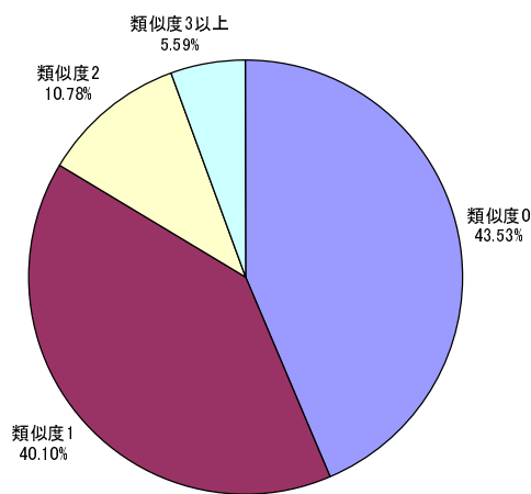
(a) 次元数 14
