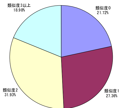
(b) 次元数 42
