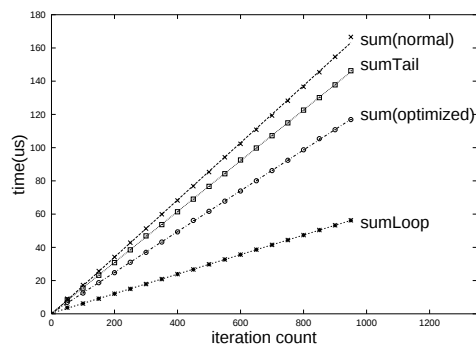
図 5 再帰回数と処理時間の関係
