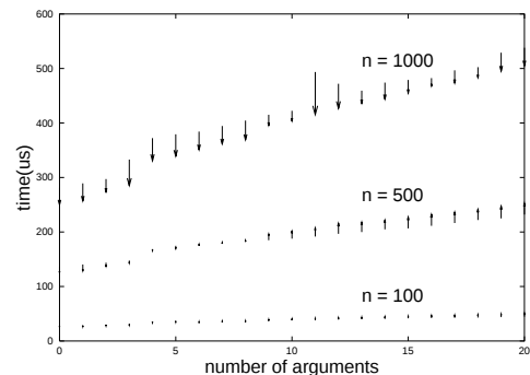
図 9 (非自己) 末尾再帰の最適化効果 (n = 100, 500, 1000)
