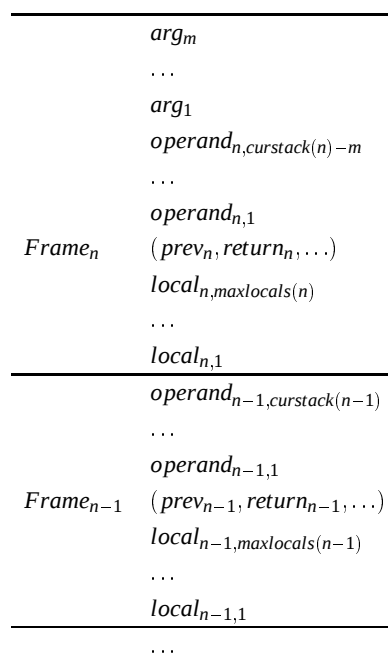
図 1 メソッド呼び出し前のフレーム状態
