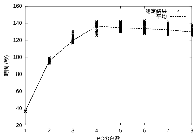
図 11: PC の台数に対する計算時間
