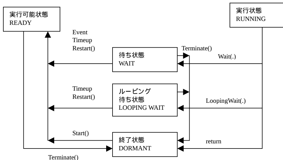
図 1 1 k-uOS, ClVrfyThrd タスク状態遷移
