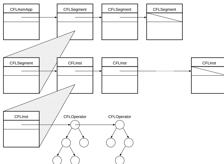
図 3: 中間表現
