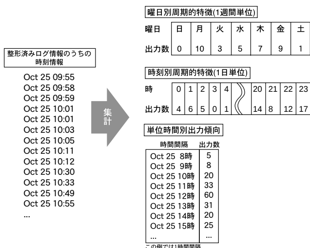
図 5: 時刻情報に基づく特徴情報の抽出
