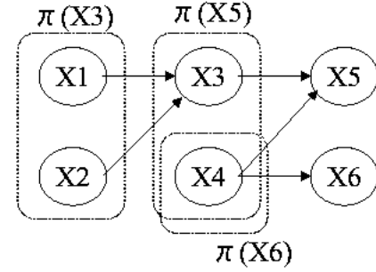
図 1: ベイジアンネットワークの例
