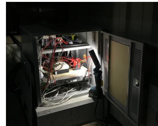
事業所屋内に設置した充放電器
