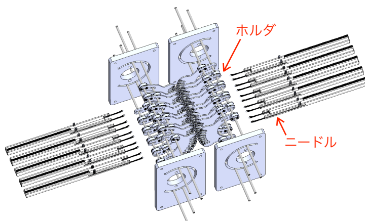
図4 ソリッド編み機の簡易図
