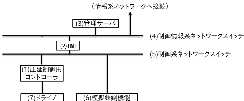
図1 鉄鋼圧延システムのシステム構成図
