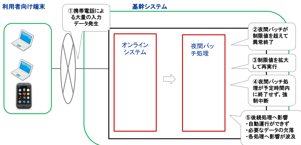
図 3. 18 - 1 障害の経緯
