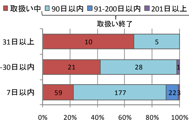
図13. 脆弱性情報の通知に要した日数別の取扱い状況
