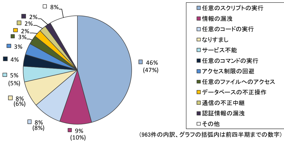
図1-6.ソフトウェア製品の脆弱性の脅威別内訳 (届出受付開始から2010年9月末まで)
