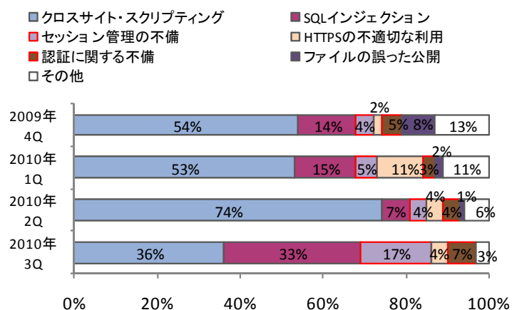
図8.四半期別脆弱性の種類別届出割合
