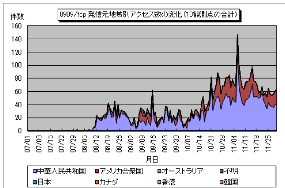
図 1-3 : 8909/tcp 発信元地域別アクセス数の変化 (10 観測点の合計)
