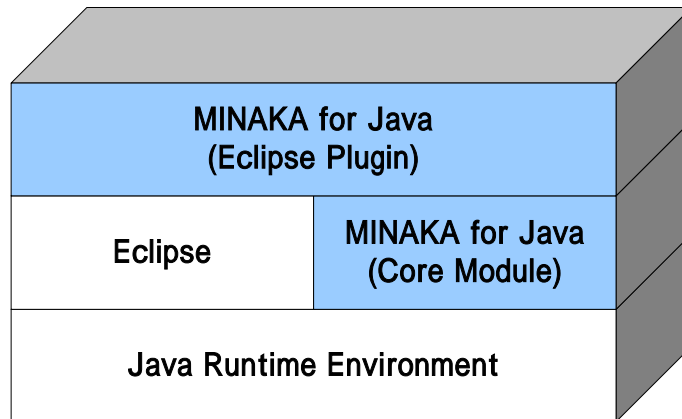
図 2 「MINAKA for Java」の実行環境
